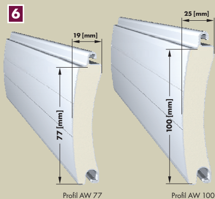
Dwa rodzaje profili
